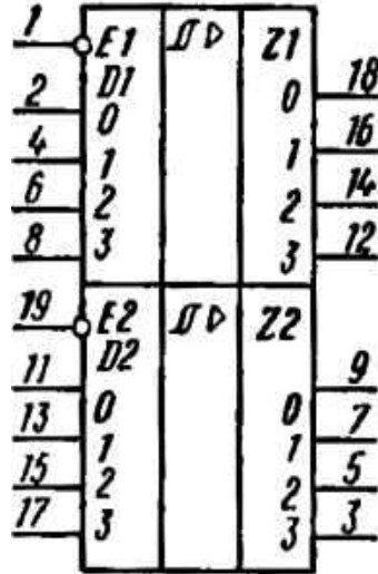
Условное графическое обозначение К555АП5
