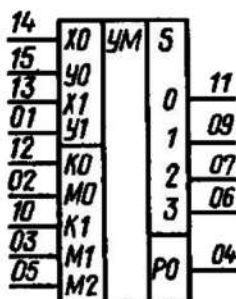
Условное графическое обозначение К561ИП5
