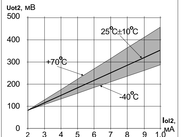
Зависимость выходного напряжения по выводу MODEOUT от тока нагрузки и температуры
