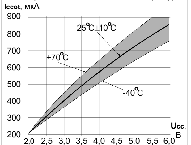
Зависимость динамического тока потребления при частотном наборе от напряжения питания и температуры
