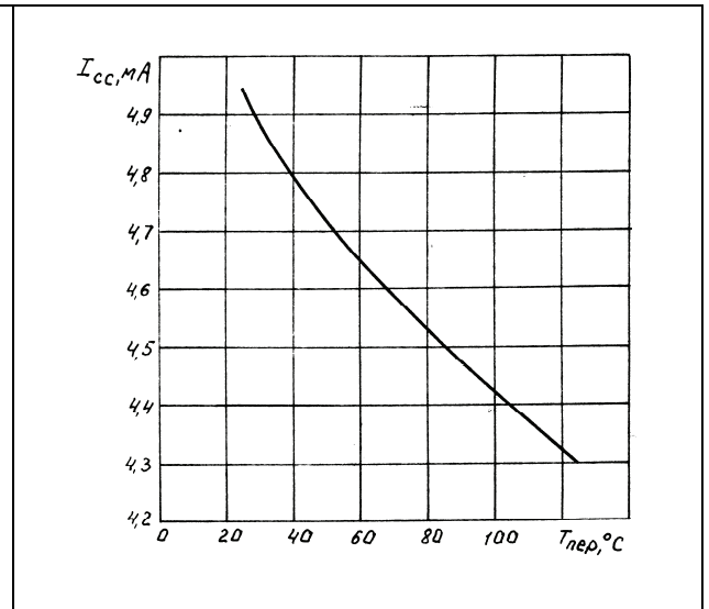
Рисунок 6. Типовая зависимость тока потребления от температуры перехода при U_i = 33 В, I_o = -40 мА для КР1181ЕН24
