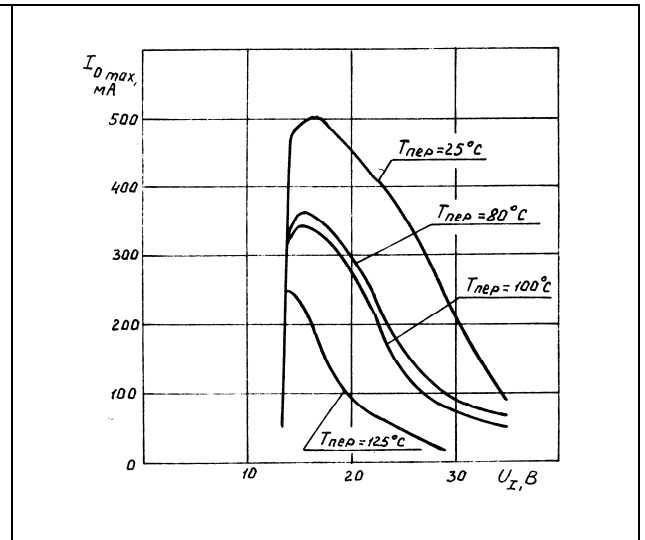
Рисунок 8. Типовая зависимость максимального выходного тока от входного напряжения при заданной температуре перехода для КР1181ЕН12
