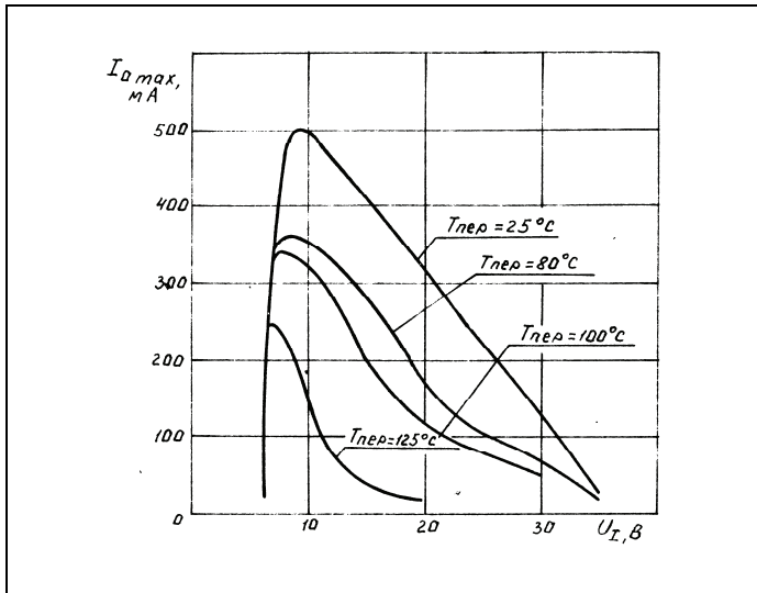
Рисунок 7. Типовая зависимость максимального выходного тока от входного напряжения при заданной температуре перехода для КР1181ЕН5
