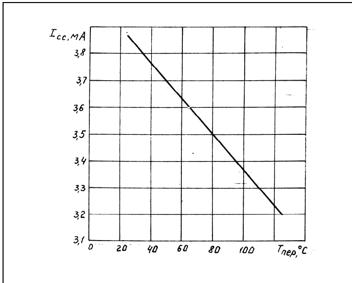
Рисунок 5. Типовая зависимость тока потребления от температуры перехода при U_i = 19 В, I_o = -40 мА для КР1181ЕН12
