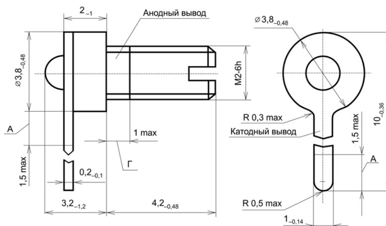
Габаритный чертеж диодов
