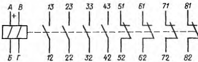
Рис. 3-38. Конструктивные данные и принципиальная электрическая схема реле РПС56
