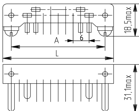
Рисунок 4 Розетка двухрядная
