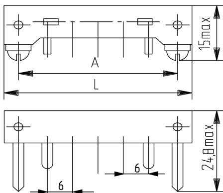
Рисунок 2 Розетка однорядная
