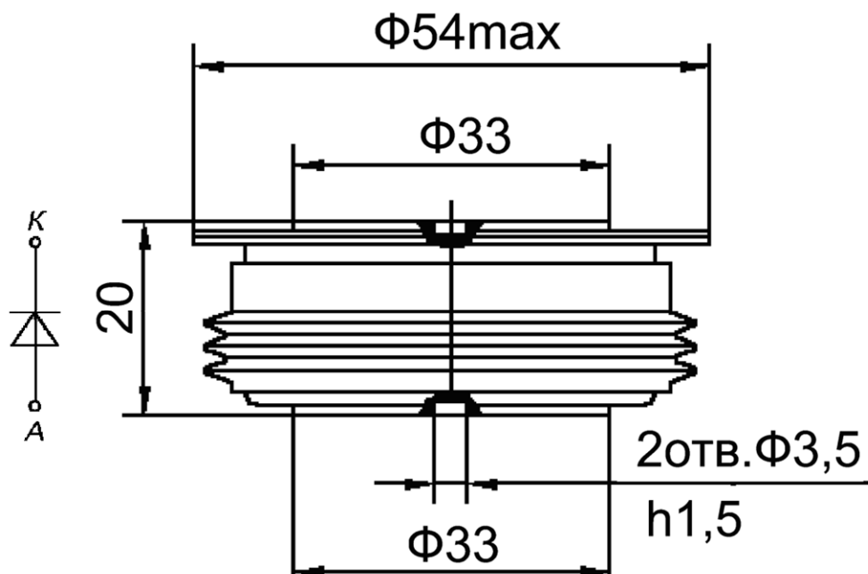
Рис. 11. Габаритные и установочные размеры
