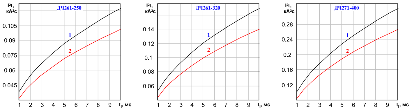
Рисунок 5: Зависимость защитного показателя I^2t от длительности импульса тока t_1 при исходной температуре структуры T_j=25^\circ\text{C} (1) и максимально допустимой температуре перехода T_{jm} (2).
