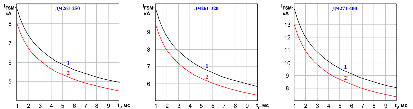
Рисунок 4: Зависимость допустимой амплитуды ударного прямого тока I_{FSM} от длительности импульса тока t_p при исходной температуре структуры T_j=25^\circ\text{C} (1) и максимально допустимой температуре перехода T_{jm} (2).
