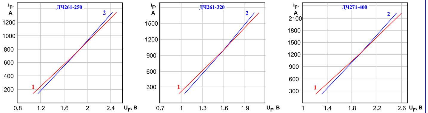
Рисунок 1: Пределные вольтамперные характеристики при максимально допустимой температуре перехода T_{jm} (1) и температуре T_j=25^\circ\text{C} (2), I_F=3,14 I_{F(AV)} .
