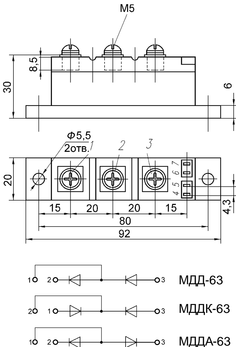
Рис. 11. Габаритные и установочные размеры
