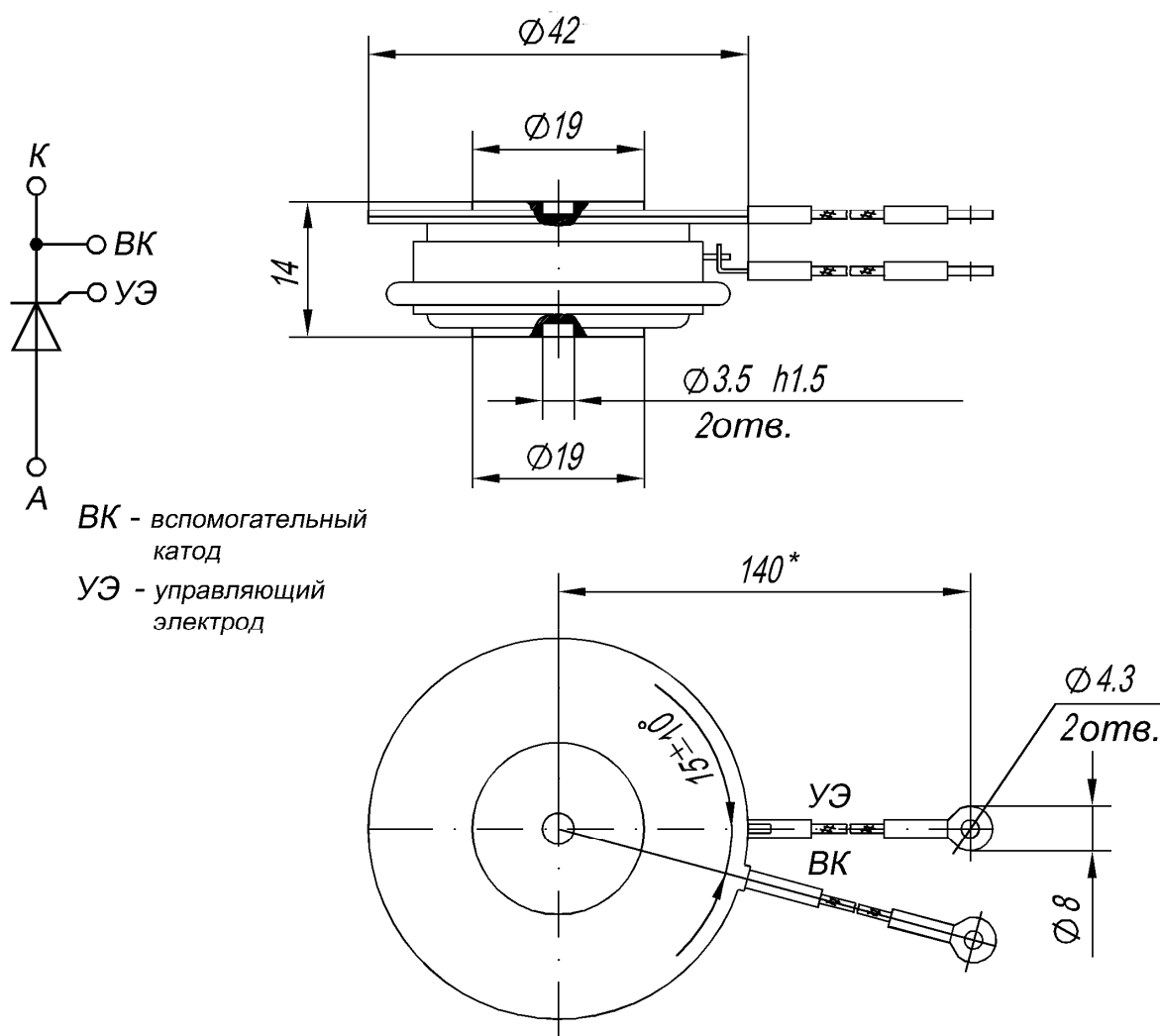
Рис. 12. Габаритные и установочные размеры
