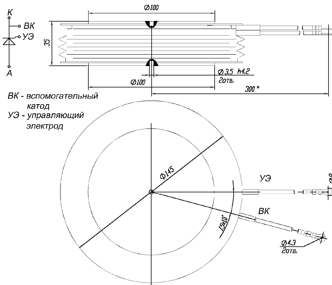
Рис. 12. Габаритные и установочные размеры
