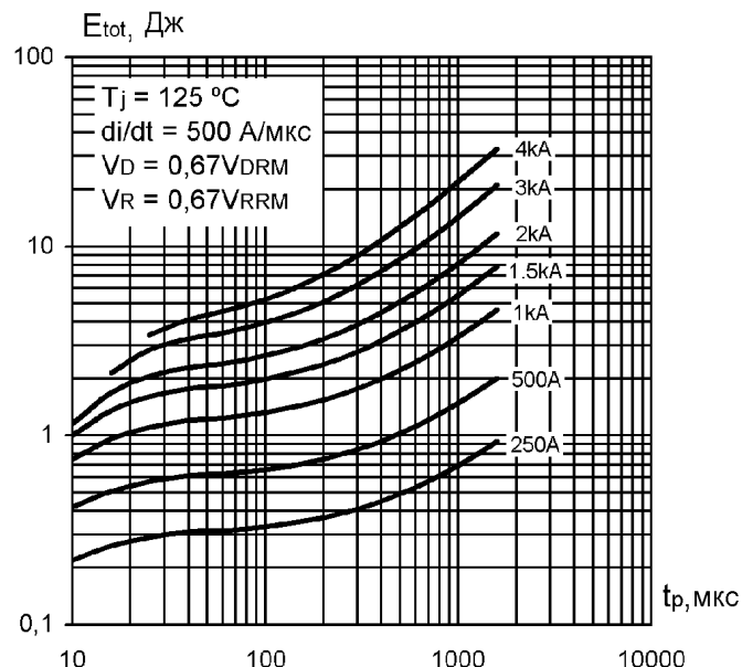
Рис. 27. Суммарная энергия потерь одного трапецидального импульса тока
