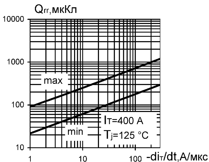
Рис. 8. Зависимость заряда обратного восстановления от скорости спада тока
