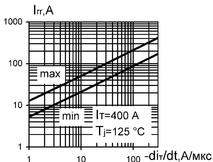
Рис. 9. Зависимость тока обратного восстановления от скорости спада тока
