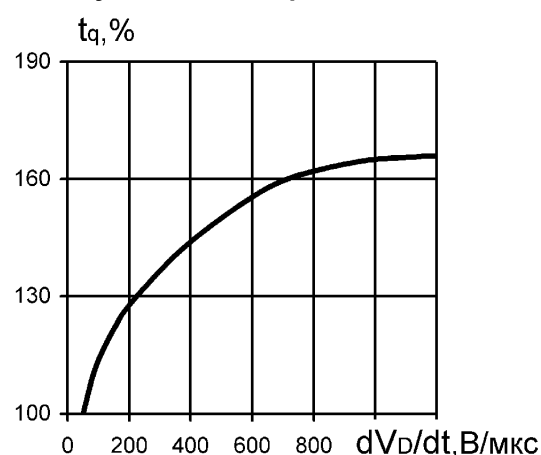
Рис. 18. Зависимость времени выключения от скорости нарастания напряжения в закрытом состоянии
