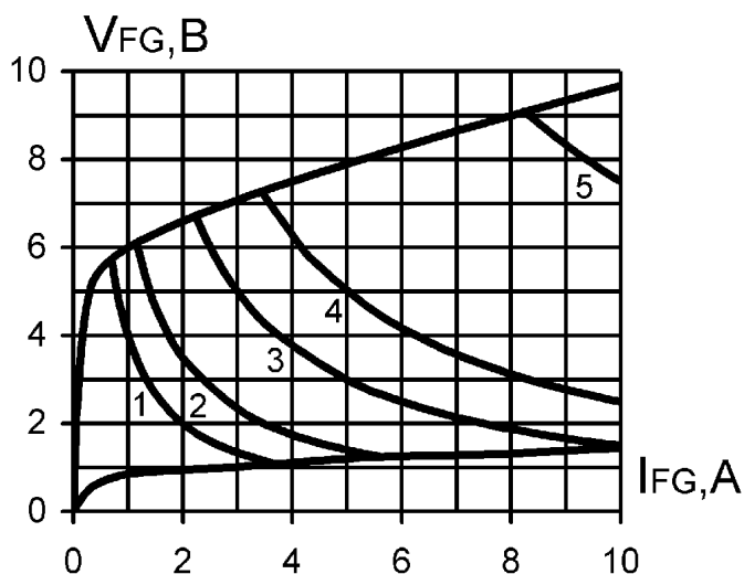
Рис. 10. Предельные характеристики цепи управления
