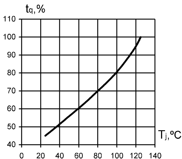
Рис. 12. Зависимость времени выключения от температуры перехода
