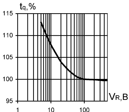
Рис. 15. Зависимость времени выключения от обратного напряжения
