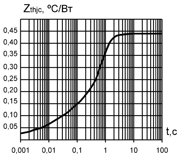
Рис. 2. Переходное тепловое сопротивление переход-корпус
