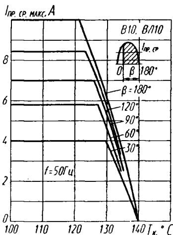
Зависимости допустимого прямого тока от температуры
