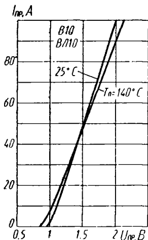
Зависимости прямого тока от напряжения
