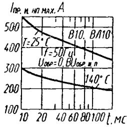
Зависимости допустимого неповторяющегося импульсного тока от времени
