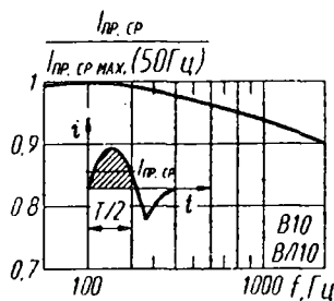
Зависимость допустимого прямого тока от частоты
