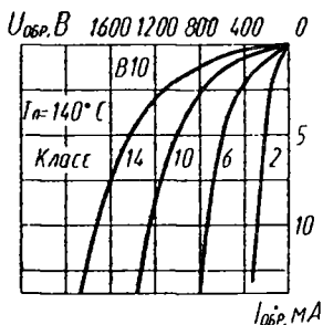
Зависимости обратного напряжения от тока
