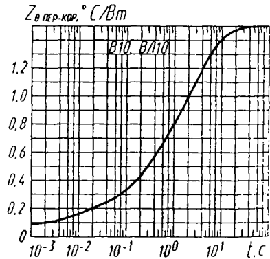
Зависимость переходного теплового сопротивления переход-корпус от времени
