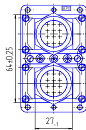
Розетка СНП337 с кожухом
