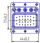
Розетка СНП336 с кожухом
