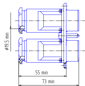
Розетка СНП337 с кожухом
