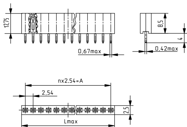
Рисунок 5 Розетка СНП346 (однорядная)
