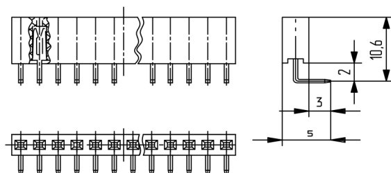
Рисунок 5а Остальное см. рисунок 5
