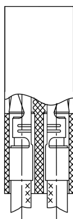
Схема установки контакта с обжатым проводом в изолятор
