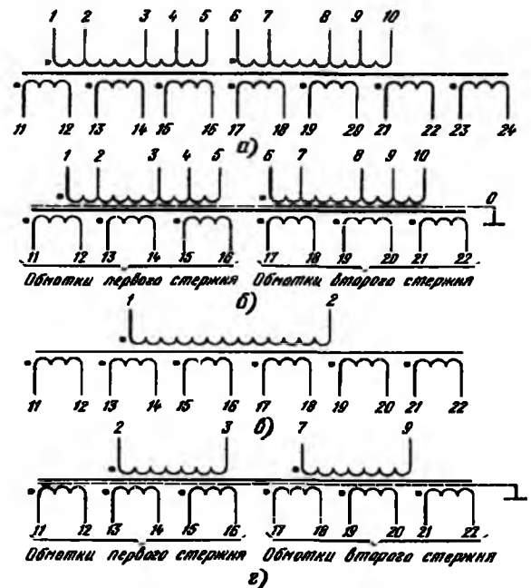
Рис. 2.10. Электрические схемы трансформаторов типа ТПП с частотой питающей сети 50 Гц: а — броневой конструкции с напряжением 127/220 В; б — стержневой конструкции с напряжением 127/220 В; в — броневой конструкции с напряжением 220 В; г — стержневой конструкции с напряжением 220 В
