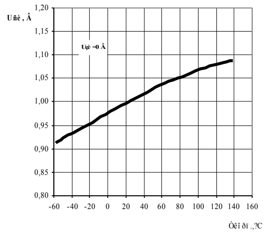
Рисунок 5 - Зависимость нормализованного напряжения сток-исток U_{си} от температуры корпуса T_{корп.} транзисторов 2П829И9
