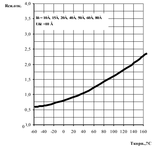
Рисунок 4 - Зависимость нормализованного сопротивления сток-исток в открытом состоянии R_{си.отк.} от температуры корпуса T_{корп.} транзисторов 2П829И9
