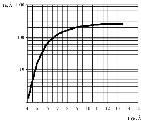
Рисунок 2 - Зависимость тока стока I_c от напряжения сток-исток U_{си} транзисторов 2П829И9
