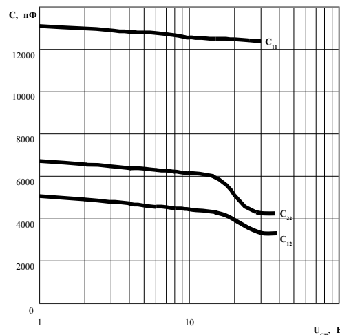
Рисунок 6 - Зависимости входной ( C_{11} ), выходной ( C_{22} ) и проходной ( C_{12} ) емкостей от напряжения сток-исток при температуре корпуса (25 \pm 10)^\circ\text{C} транзисторов 2П829И9
