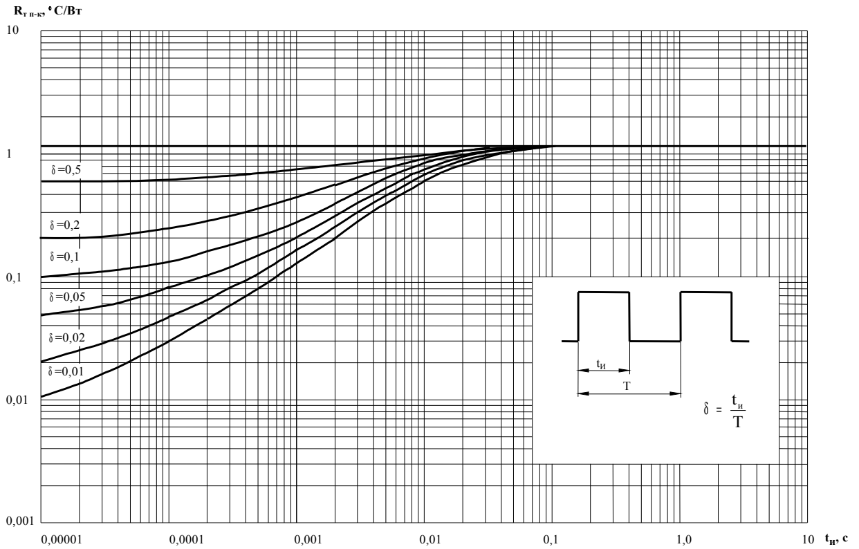
Рисунок 7– Зависимость теплового сопротивления переход-корпус R_{Tj-K} от длительности импульса t_{и} и скважности импульса \delta транзисторов 2П829И9
