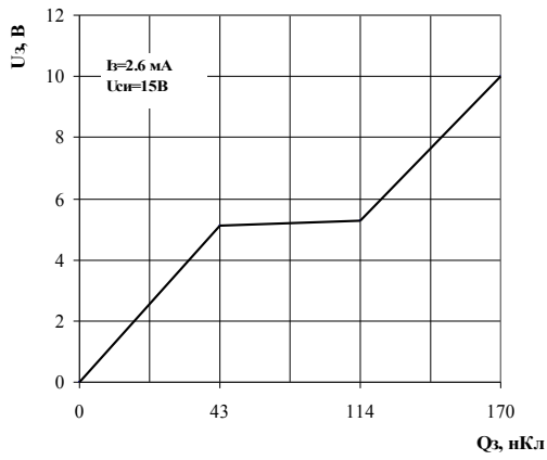
Рисунок 1 - Зависимость заряда затвора Q_z от напряжения затвора U_z для транзистора типа 2П829И9
