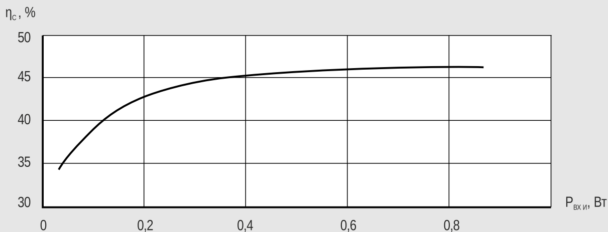
Рисунок 5. Типовая зависимость коэффициента полезного действия стока от входной импульсной мощности при U_n = 50 В и t_k \leq 40 °С, f = 1550 МГц
