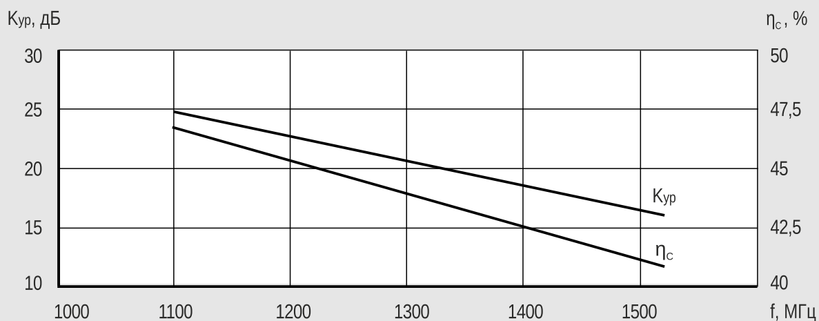
Рисунок 6. Типовые зависимости коэффициента усиления по мощности и КПД стока от частоты при P_{вх.и} = \text{const} , U_n = 50 В, t_k \leq 40 °С
