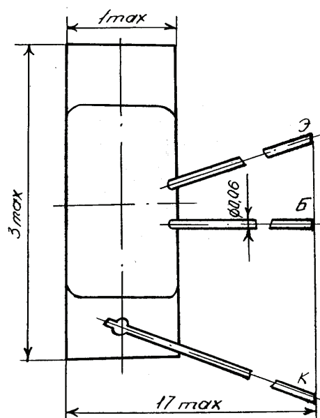
Транзистор КТ625АМ-2 Масса не более 0,004 г
