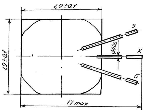
Транзистор КТ625А-2 Масса не более 0,015 г
