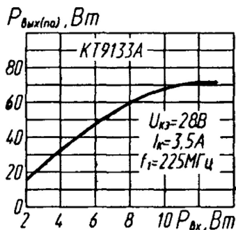
Зависимость выходной мощности от входной
