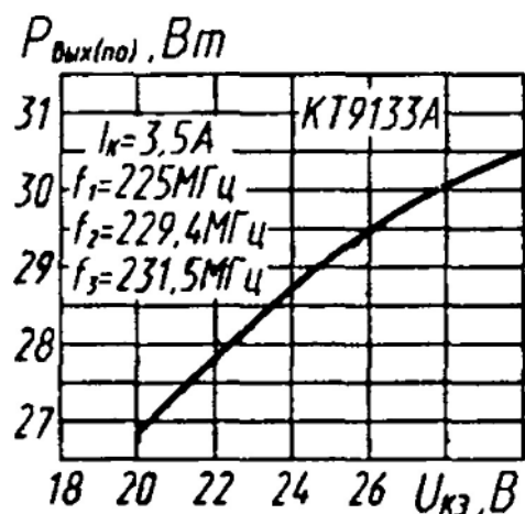
Зависимость выходной мощности от напряжения коллектор—эмиттер
