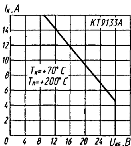
Зависимость тока коллектора от напряжения коллектор—база
