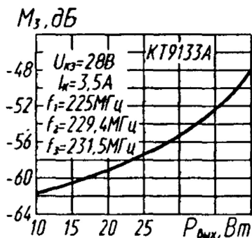
Зависимость коэффициента комбинационных составляющих третьего порядка от выходной мощности
