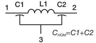
Вариант 3 - Pi-фильтр (фильтр индуктивно-емкостной, трехэлементный): I_{НОМ}=15; 25 \text{ A} Б26-3
