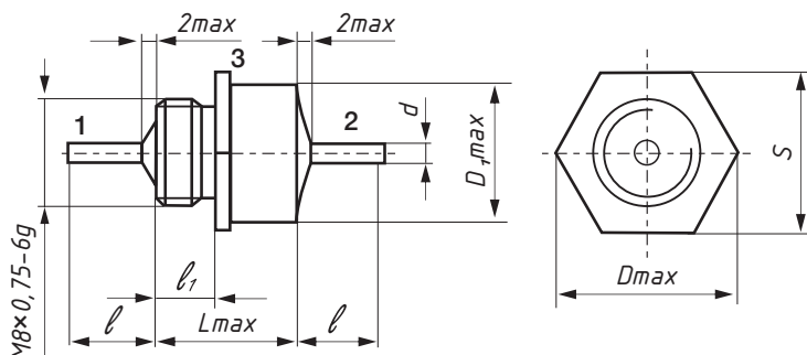
Размеры и масса фильтров. Размеры в миллиметрах
