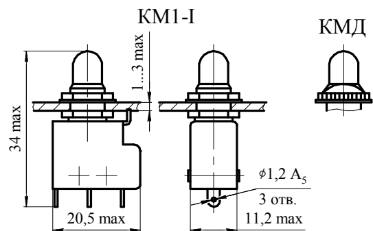
Габаритные и установочные размеры
