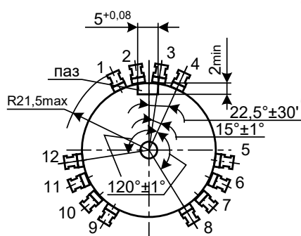
Общий вид потенциометра ПТ1-6А
