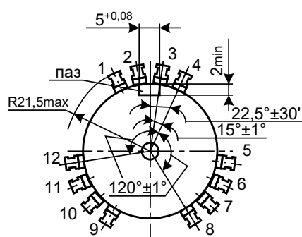
Общий вид потенциометра ПТ1-6Б
