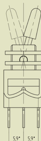
ПТ503-2, ПТ504-2 (остальное см. ПТ503-1, ПТ504-1)
