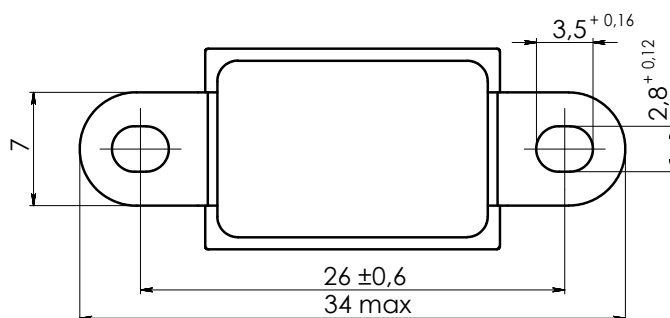
Исполнение 2 для навесного монтажа
