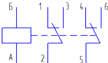
Порядок расположения выводов контактов и обмоток
