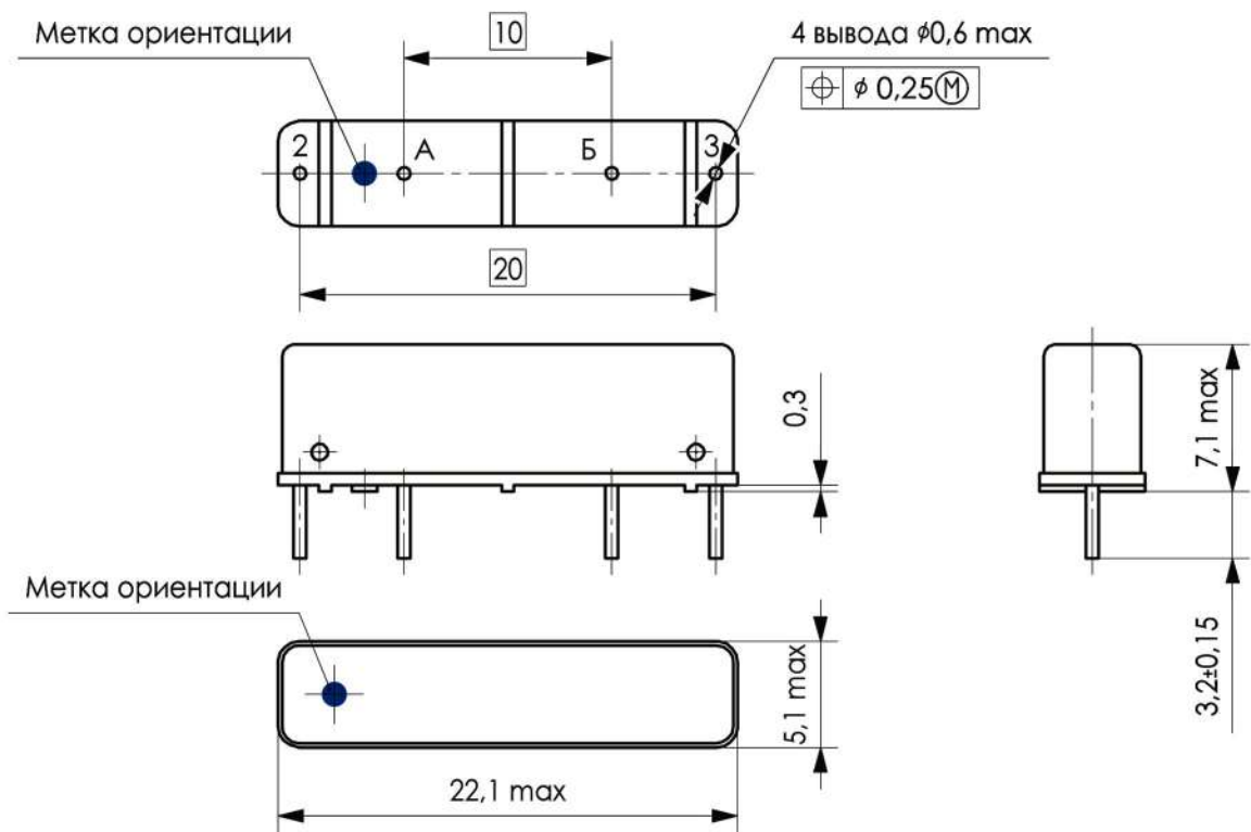
Габаритные, установочные и присоединительные размеры. Расположение выводов контактов и обмоток Исполнение РГК 36 и РГК 36В
