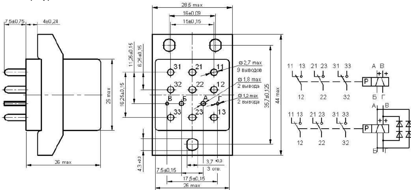
Рис. 1 – Общий вид реле РПК78 с фланцем и принципиальная электрическая схема
