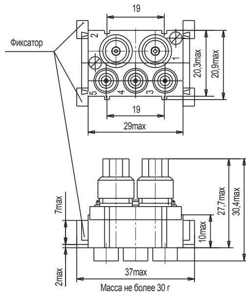
Рисунок 6 Розетка РПН23-5Г2-КД
