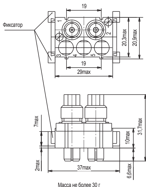
Рисунок 7 Вилка РПН23-3Ш-КД
