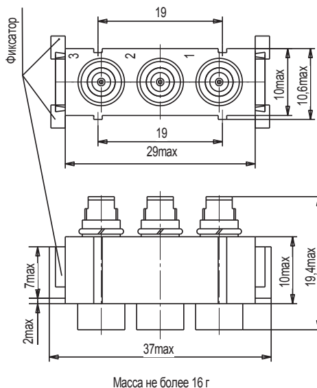
Рисунок 8 Розетка РПН23-3Г-КД
