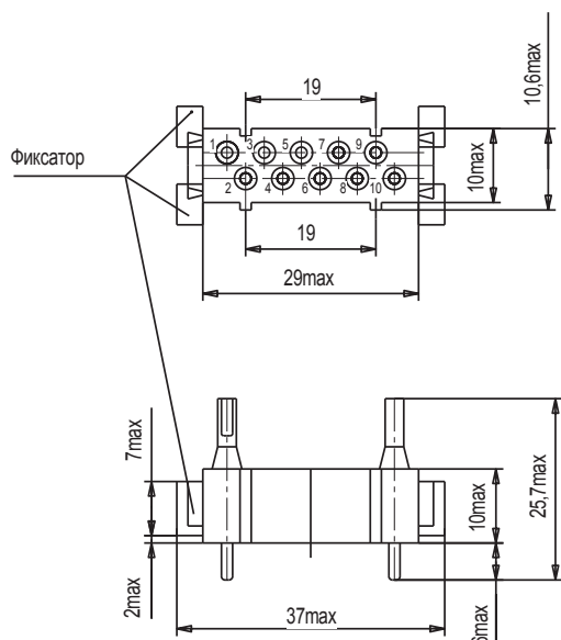
Рисунок 1 Вилка РПН23-10Ш-КД
