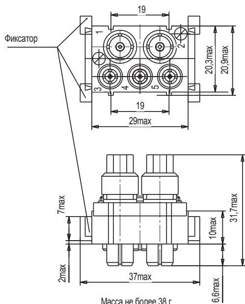
Рисунок 5 Вилка РПН23-5Ш2-КД
