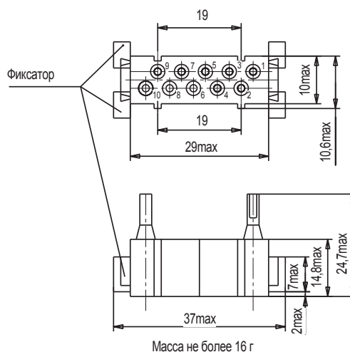
Рисунок 2 Розетка РПН23-10Г-КД
