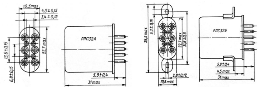
Габаритные и присоединительные размеры
