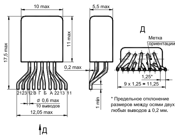
Рис. 2 - Общий вид реле РПС46-1
