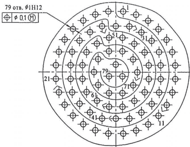
СХЕМА СНЦ144К-79/21
