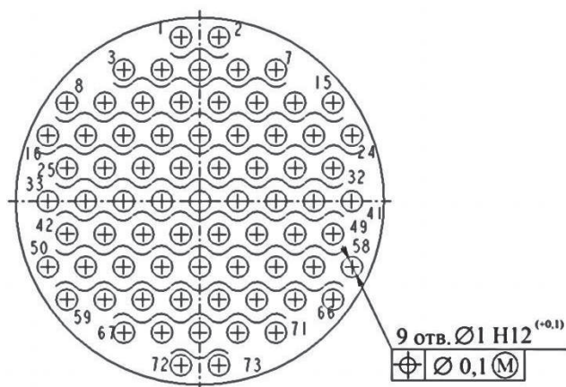
СХЕМА СНЦ144К-73/17
