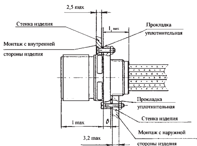
Установка приборных вилок и розеток на изделии
