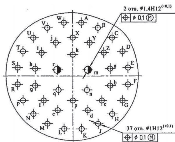
СХЕМА СНЦ144К-39/21
