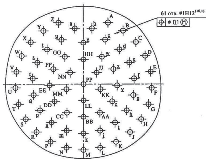
СХЕМА СНЦ144К-61/25
