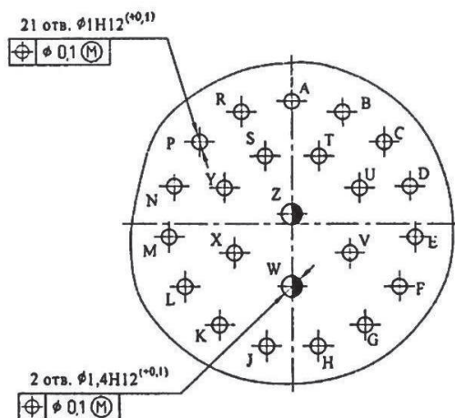
СХЕМА СНЦ144К-23/17
