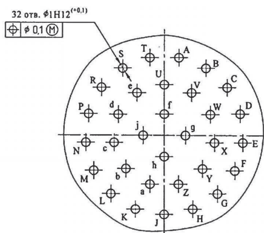
СХЕМА СНЦ144К-32/19
