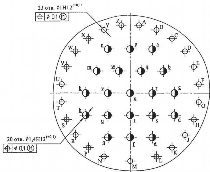
СХЕМА СНЦ144К-56/25
