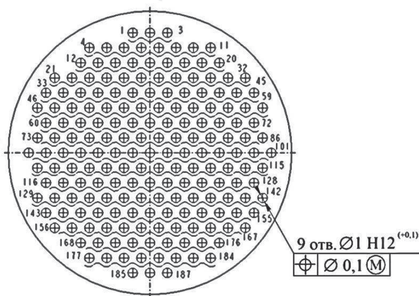
СХЕМА СНЦ144К-187/25
