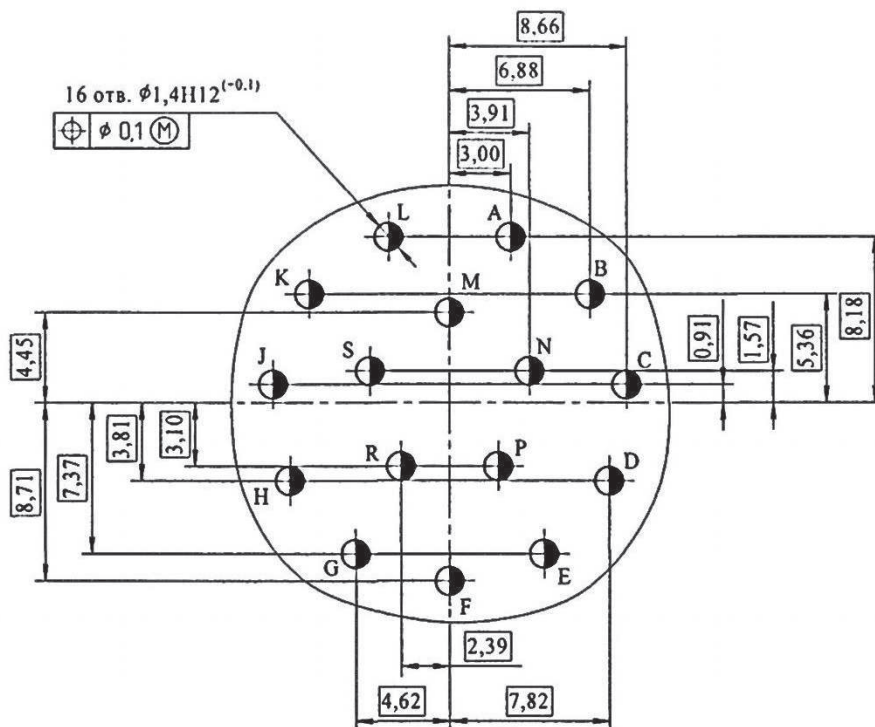
СХЕМА СНЦ144К-79/21
