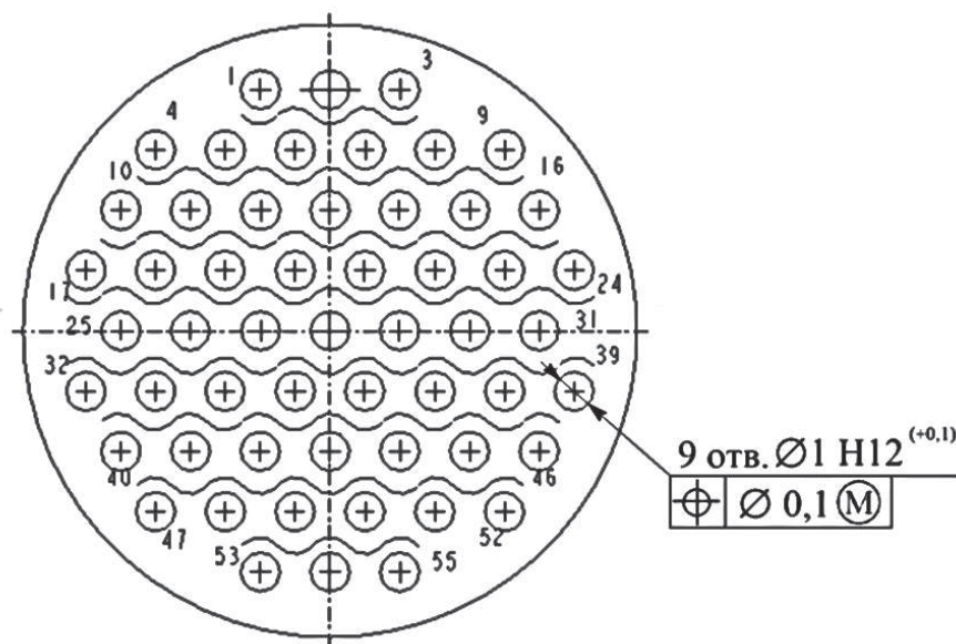
СХЕМА СНЦ144К-55/15
