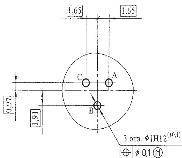
СХЕМА СНЦ144К-3/9
