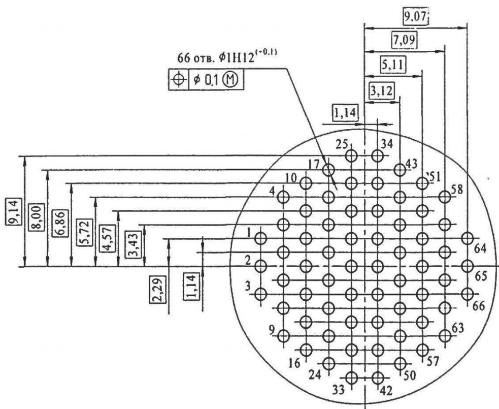
СХЕМА СНЦ144К-88/19
