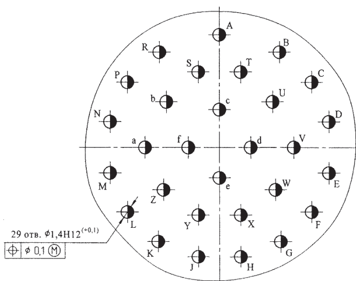
СХЕМА СНЦ144К-29/25
