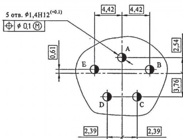
СХЕМА СНЦ144К-5/15
