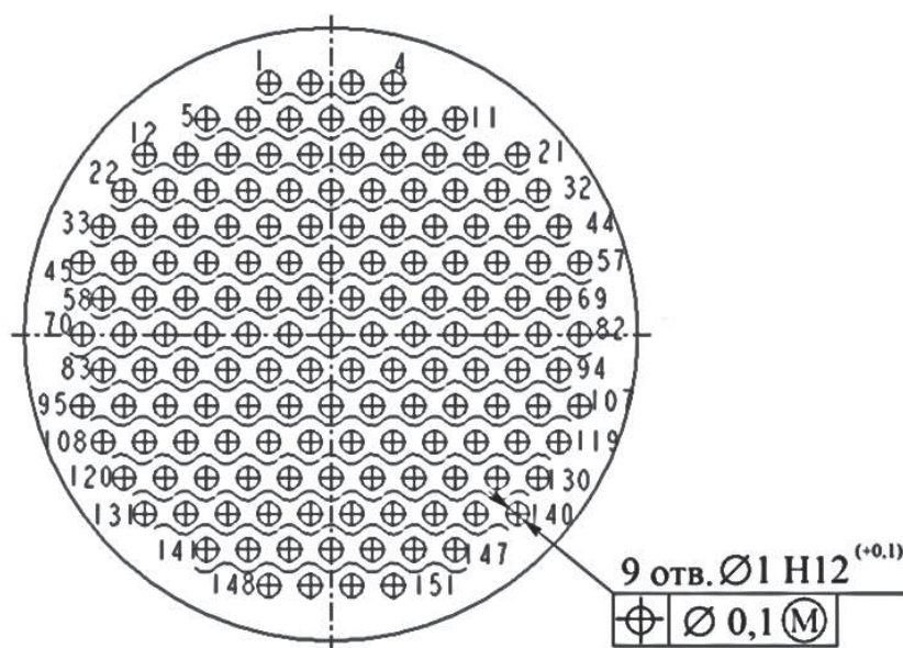
СХЕМА СНЦ144К-151/23
