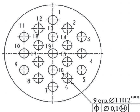
СХЕМА СНЦ144К-19/11
