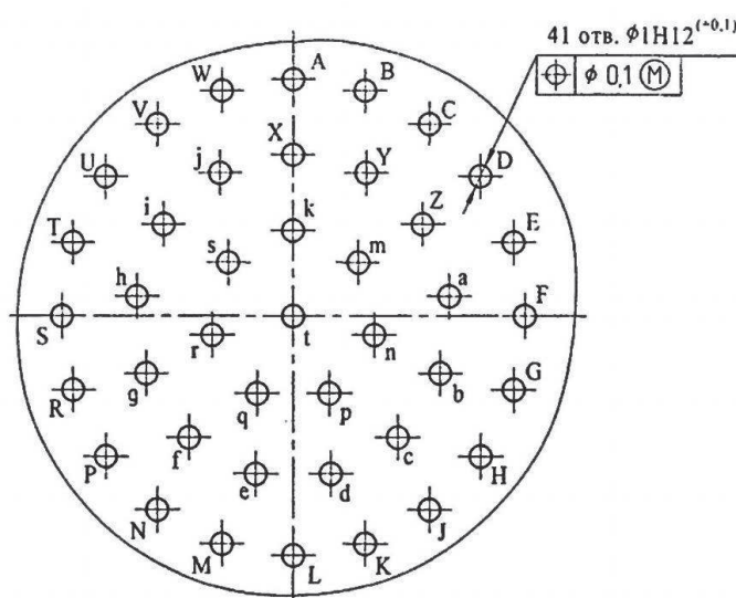
СХЕМА СНЦ144К-41/21
