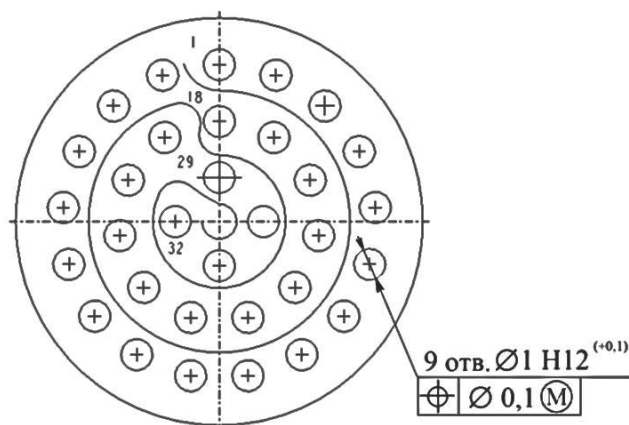
СХЕМА СНЦ144К-32/13
