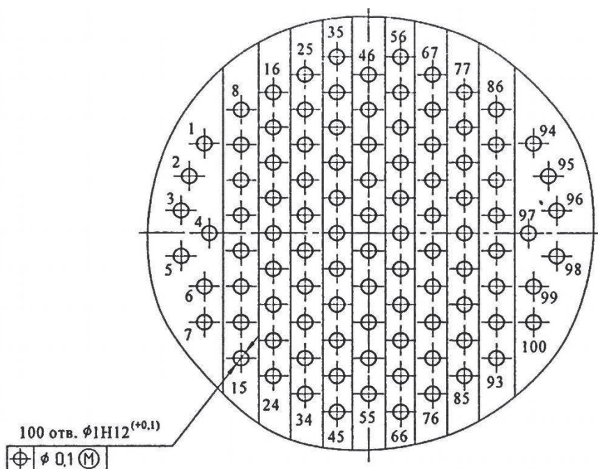
СХЕМА СНЦ144К-100/23
