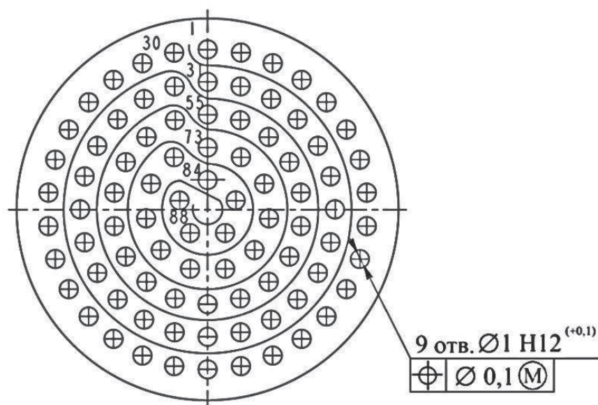
СХЕМА СНЦ144К-88/19
