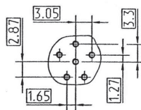
СХЕМА СНЦ146-7/14
