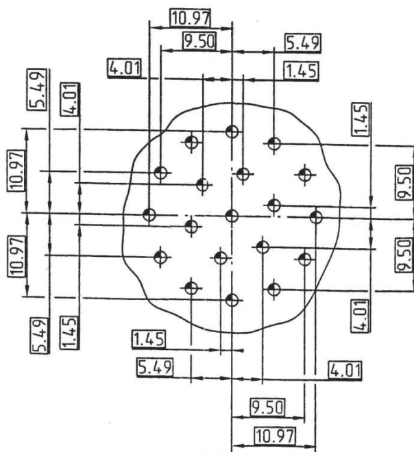
СХЕМА СНЦ146-61/24
