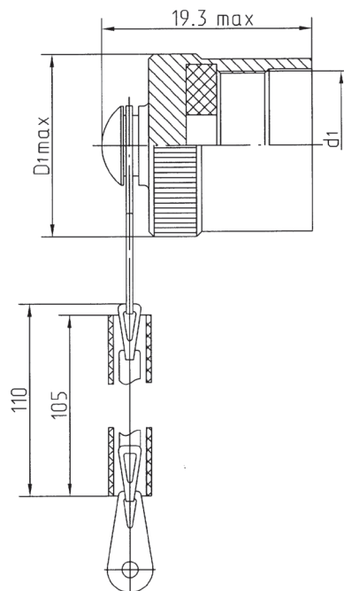
Заглушка ЭП146-3/8(10,12,14,16,18,20,22,24)
