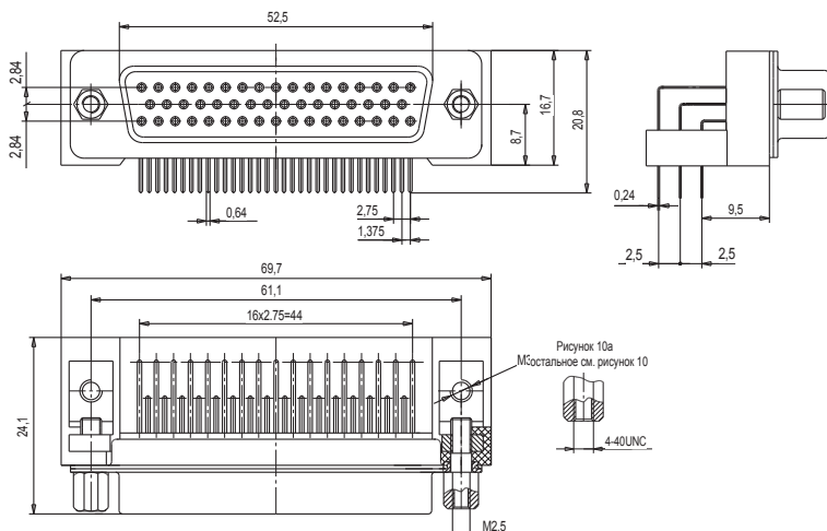
Рисунок 11 Вилки СНП268-9(15,25,37)ВП31(2)-1(3)-3(4)(-В)
