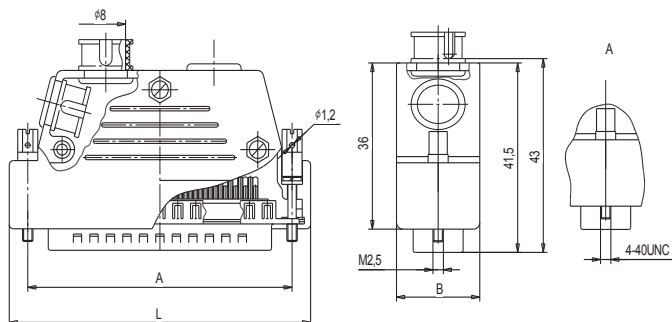
Рисунок 18 Вилки СНП268-25(37,50)ВРП11(2)5(6)-2(4)-(-В)
