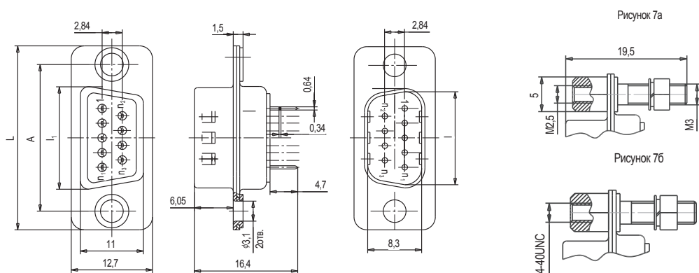
Рисунок 7 Вилки СНП268-9(15,25,37)ВП21(2)-0(1,3)(-В)
