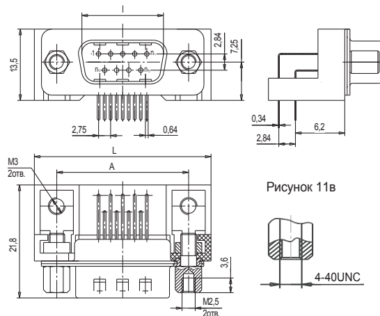
Рисунок 116 Вилки СНП268-9(15,25,37)ВП31(2)-1(3)-5(-В)
