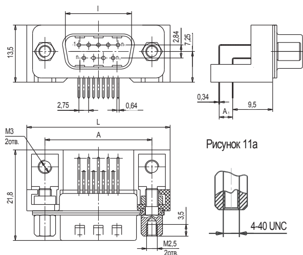
Рисунок 11 Вилки СНП268-9(15,25,37)ВП31(2)-1(3)-3(4)(-В)
