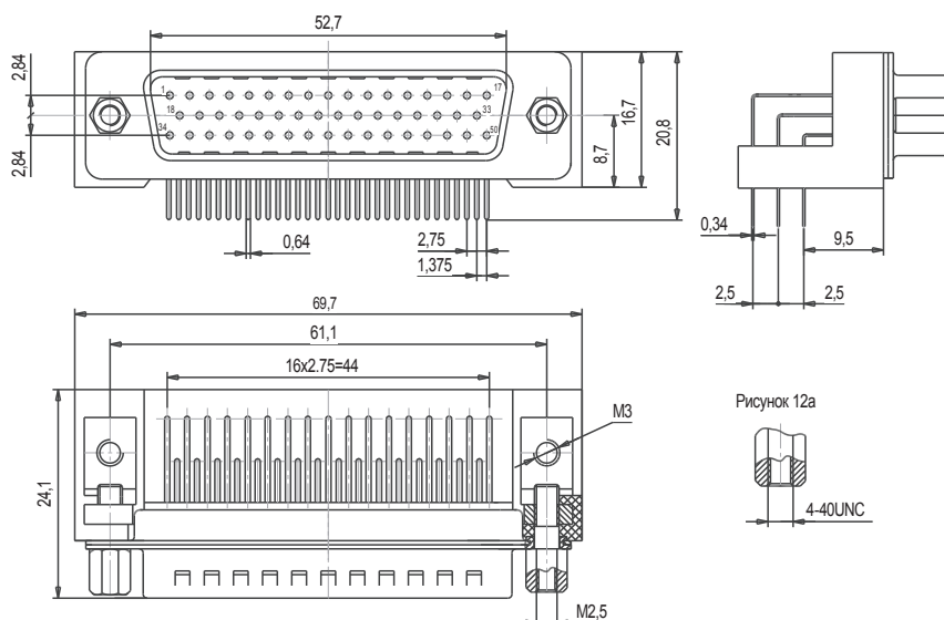
Рисунок 12 Вилки СНП268-50ВП31(2)-1(3)-4(-В)
