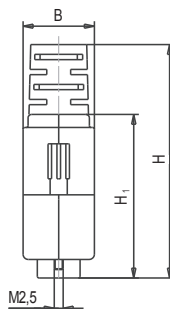
Рисунок 14 Вилки СНП268-9(15,25,37,50)ВП11(2)1(2)-1(2,3,4)-(-В)
