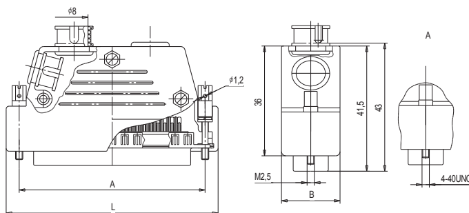
Рисунок 17 Розетки СНП268-25(37,50)РП11(2)5(6)-2(4)-(-В)
