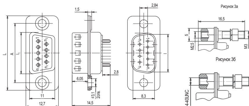
Рисунок 3 Вилки СНП268-9(15,25,37)ВП11(2)-0(1,3)(-В)
