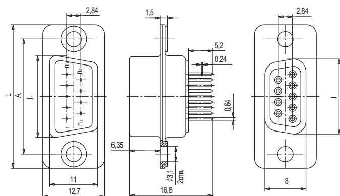
Рисунок 5 Розетки СМП268-9(15,25,37)РП21(2)-0(1,3)(-В)
