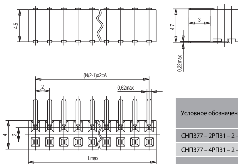
Розетка СНП377-НРП31-2-2
