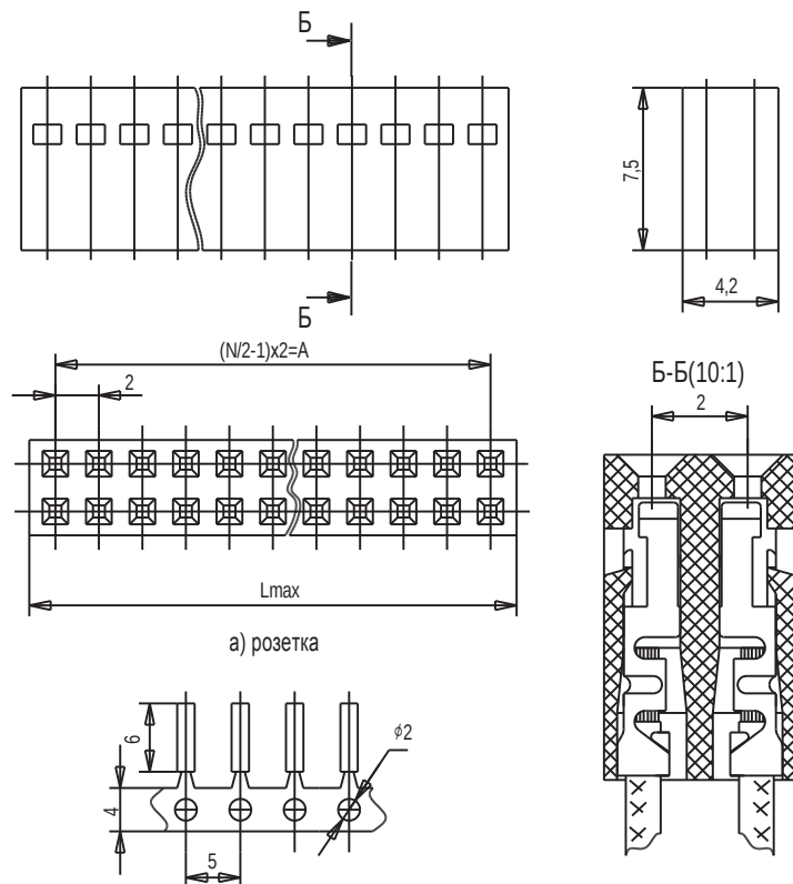
Розетка СНП377-NPO21-2
