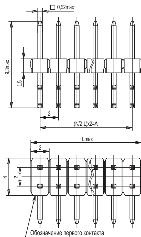
Вилка СНП377-NBП31-2
