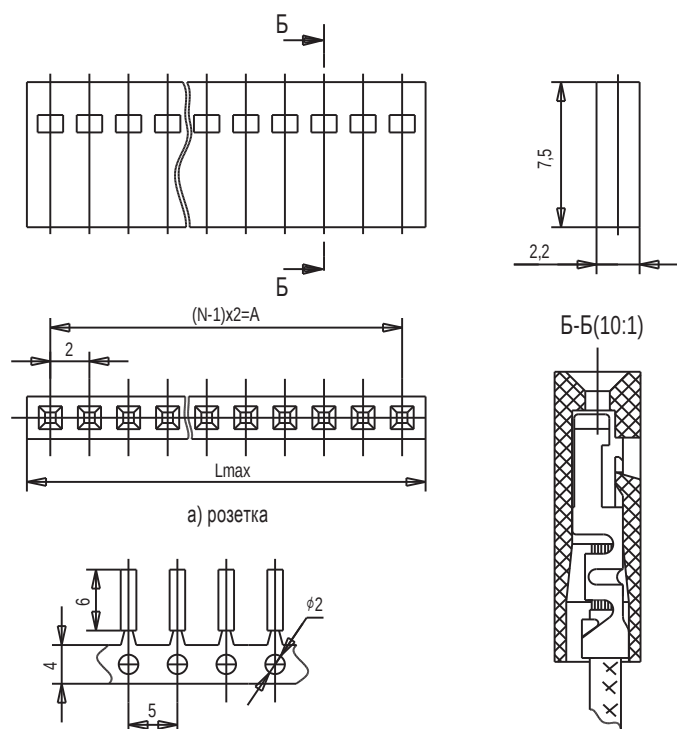
Розетка СНП377-NPO21-1
