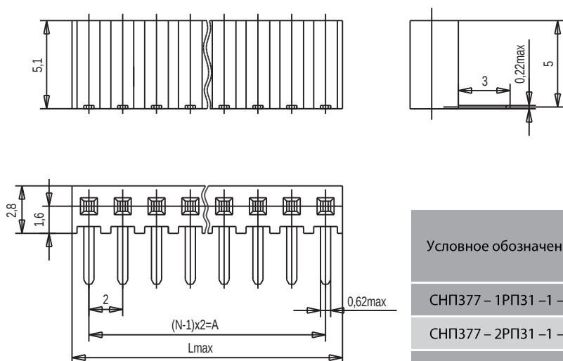
Розетка СНП377-НРП31-1-1
