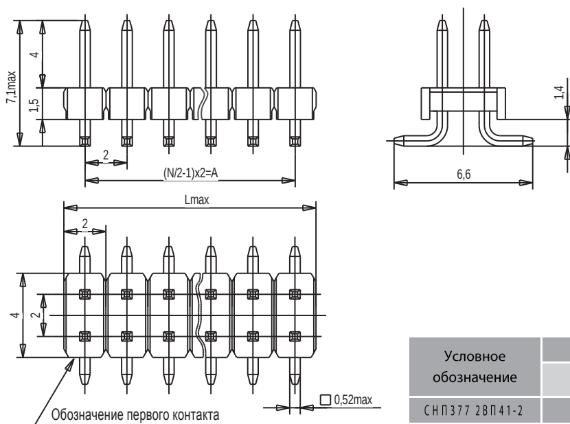
Вилка СНП377-НВП41-2
