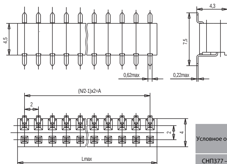
Розетка СНП377-НРП51-2
