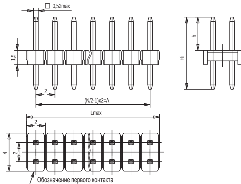
Вилка СНП377-НВП21-2-і-н
