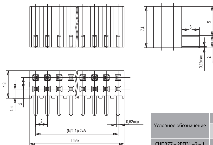
Розетка СНП377-НРП31-2-1
