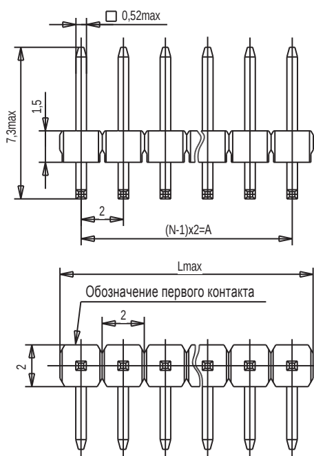
Вилка СНП377-NBП31-1
