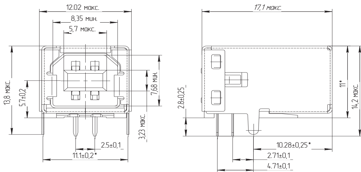
Рисунок 2 Розетка СП424-4РП31
