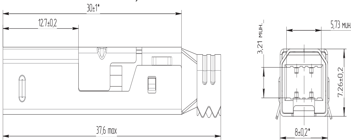
Рисунок 1 Вилка СП424-4ВП11
