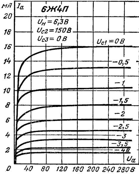
Анодные характеристики.
