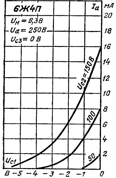
Анодно-сеточные характеристики.
