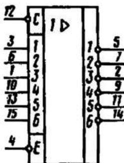
Условное графическое обозначение К564ЛН1, КФ564ЛН1В
