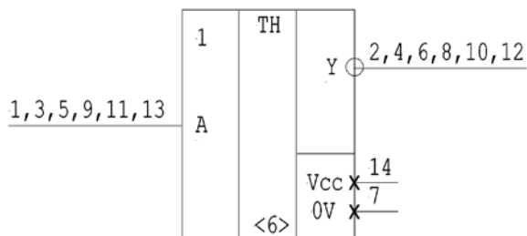
Рис. 1. Условное графическое обозначение микросхем 1564ТЛ2 ЭП в корпусе 401.14-5.
