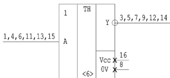
Рис. 2. Условное графическое обозначение микросхем 1564ТЛ2 ЭП в корпусе 5119.16-А.
