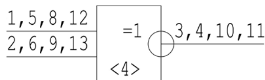
Рис. 1. Условное графическое обозначение микросхем 1564ЛП13.
