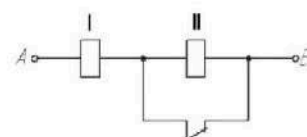
I – пусковая обмотка II – удерживающая обмотка
