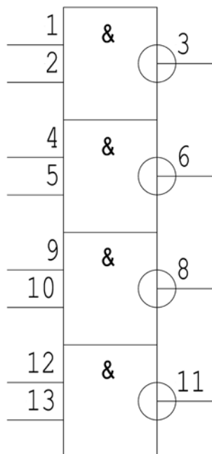
Рис. 1. Условное графическое обозначение микросхем 1564ЛА3 ЭП в корпусе 401.14-5.
