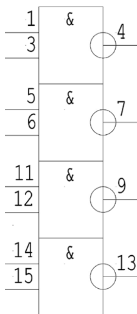
Рис. 2. Условное графическое обозначение микросхем 1564ЛА3 ЭП в корпусе 5119.16-А.
