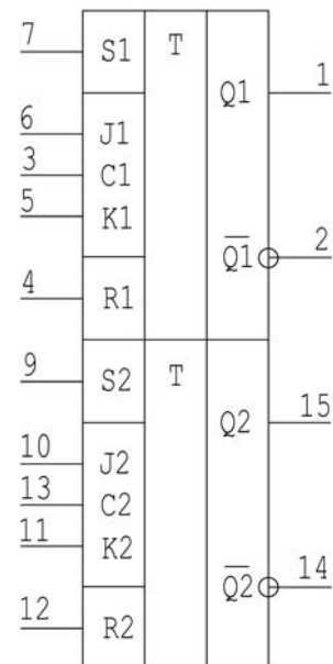
Рис. 1. Условное графическое обозначение микросхем 1526ТВ1
