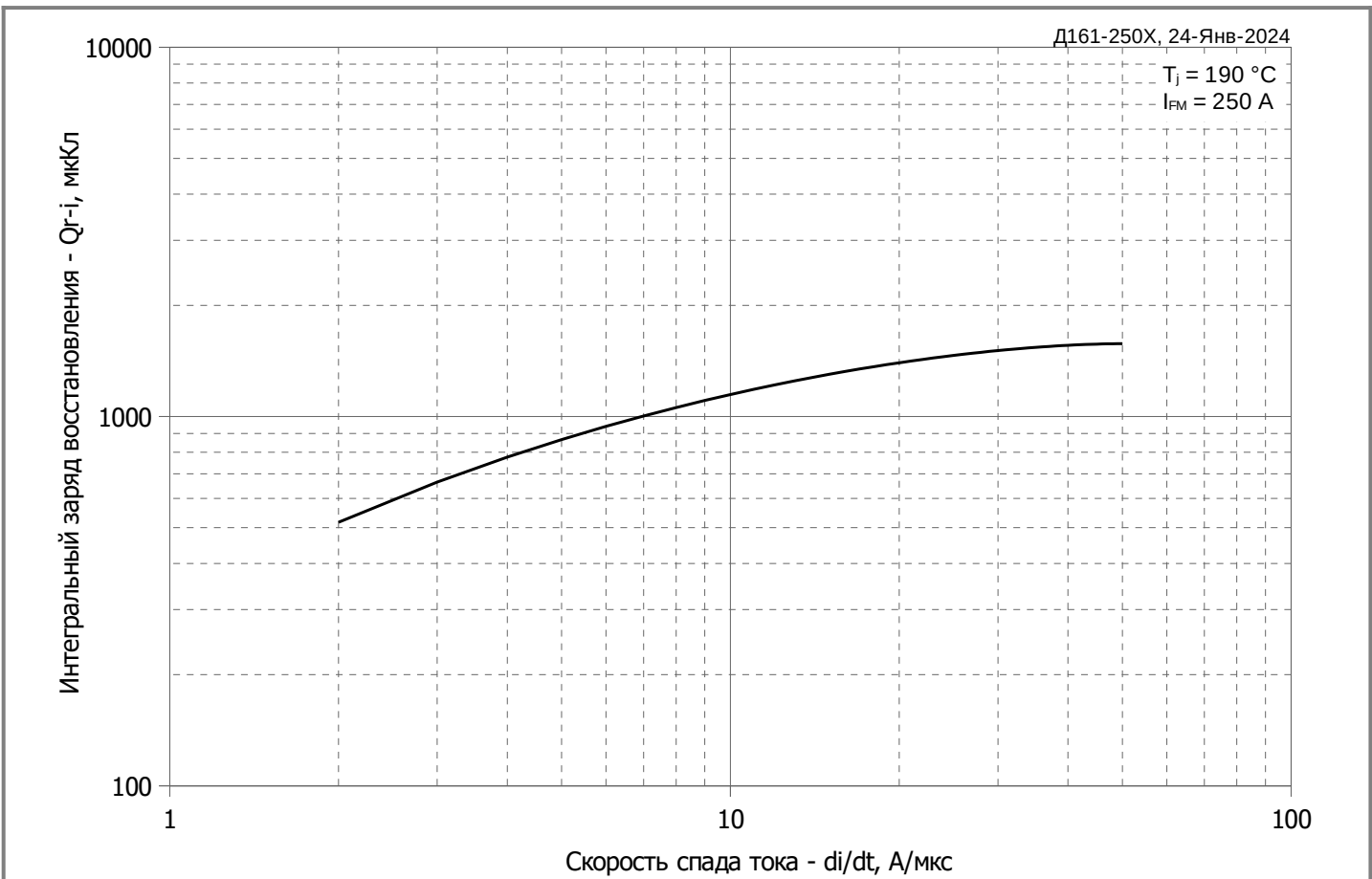
Рис. 3 – Зависимость максимального интегрального заряда обратного восстановления Q_{r-i} от скорости спада прямого тока di_R/dt
